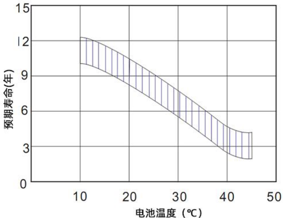
温度对长期浮充使用的影响
